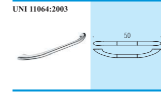
B9734 Maniglione da vasca Bath grab-bar
